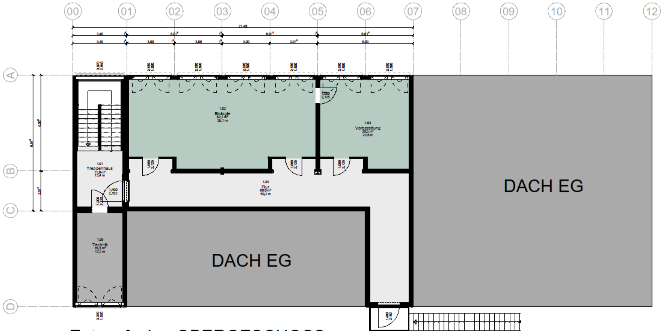
Entwurfsplan OBERGESCHOSS Variante 2
