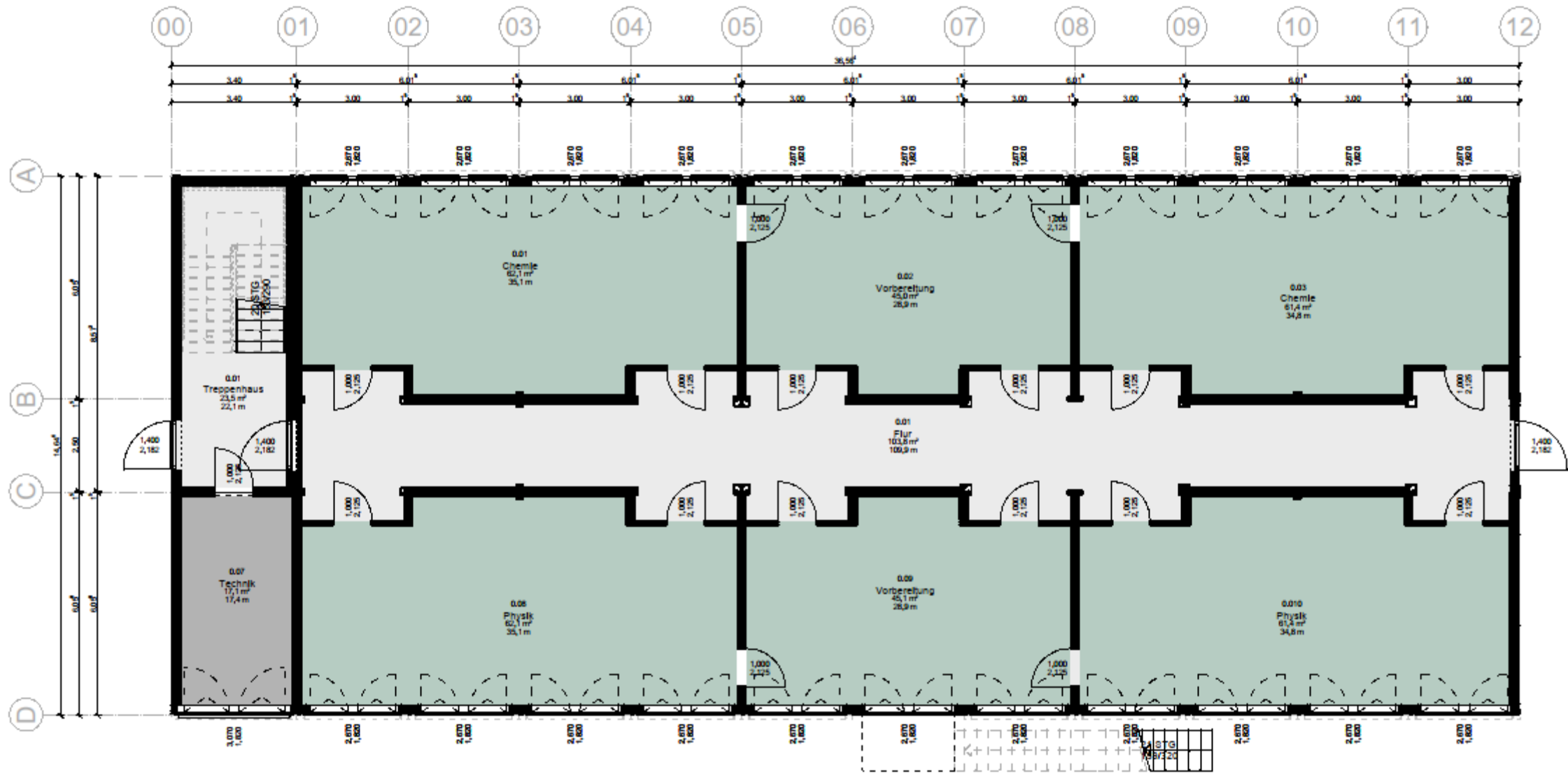
Entwurfsplan ERDGESCHOSS Variante 2
